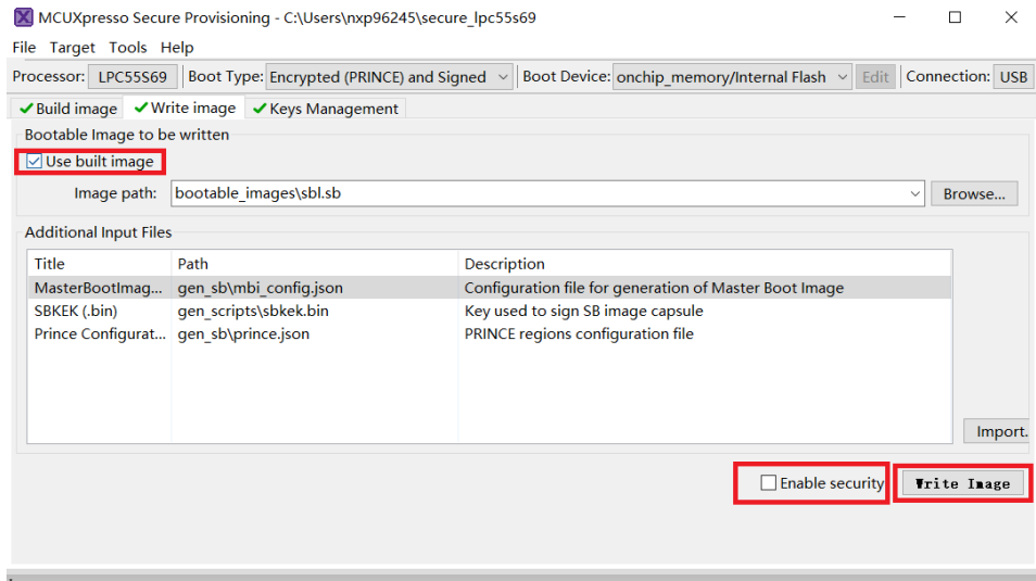
图177. 编程SBL image
