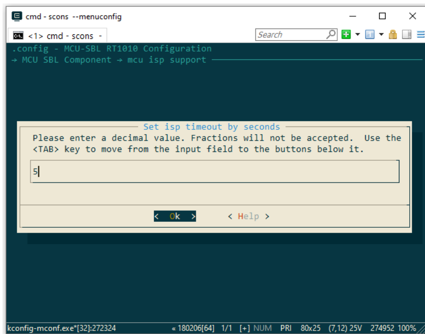
图19. SBL menuconfig 设置超时
