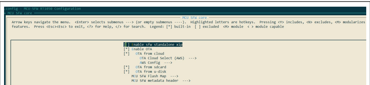
图14. SFW调试模式配置
