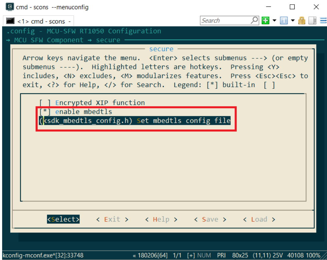
图135. 设置mbedtls配置文件
