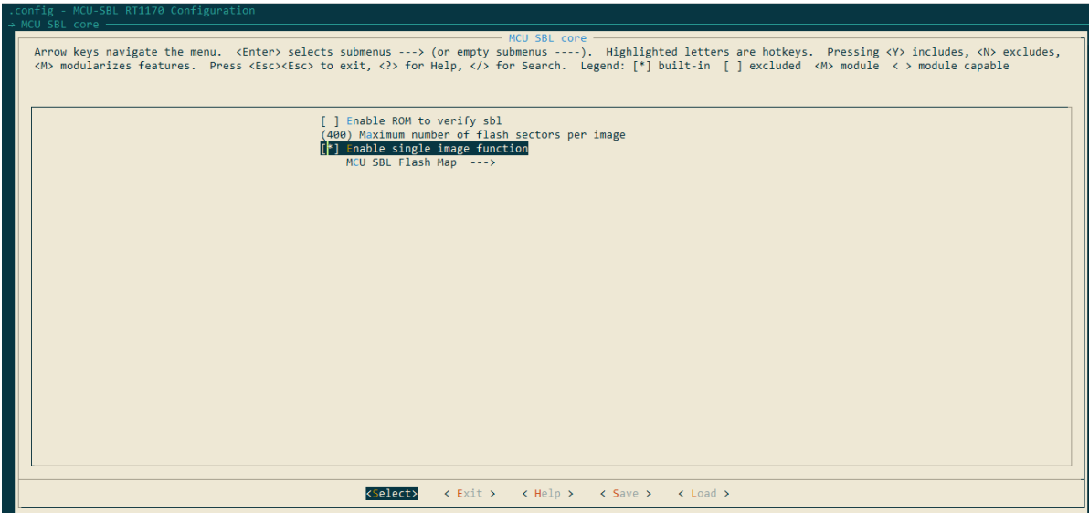
图40. 启用单一映像
