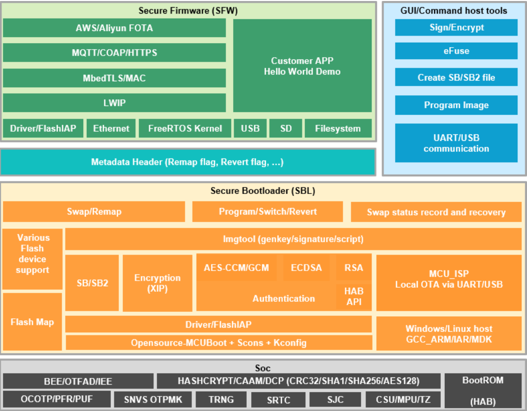
图2. MCU-OTA 项目架构
