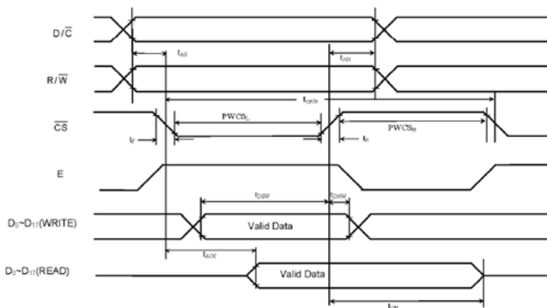
图 13. SSD1289 传输图
