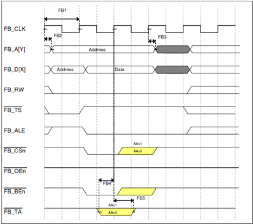
图 2. FlexBus 写周期
