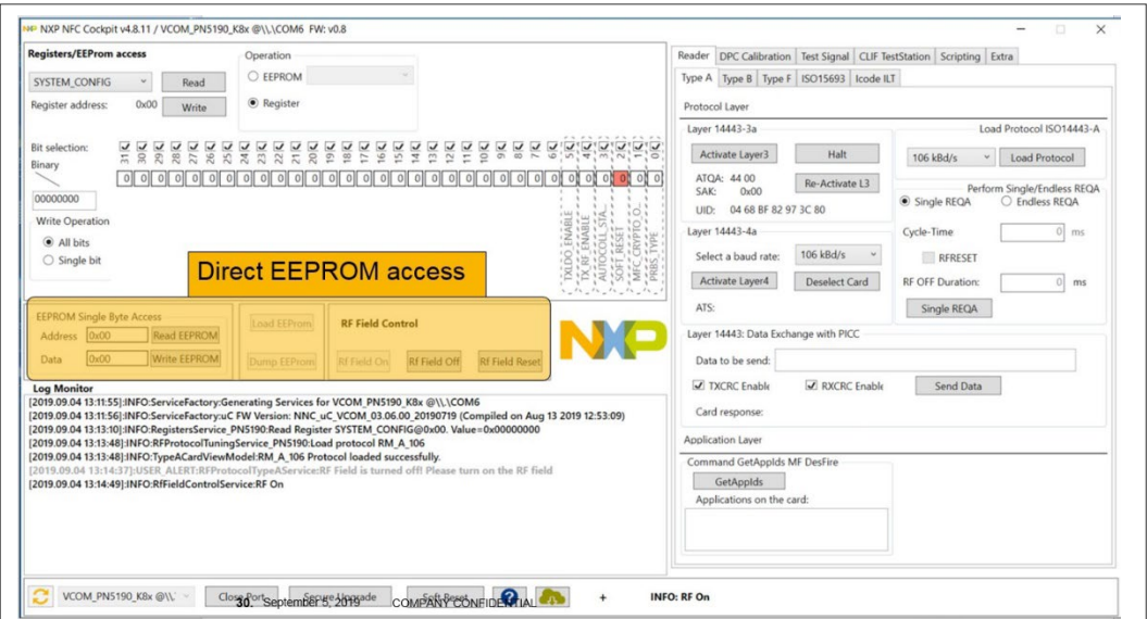
图 23. PN5190直接 EEPROM 访问
