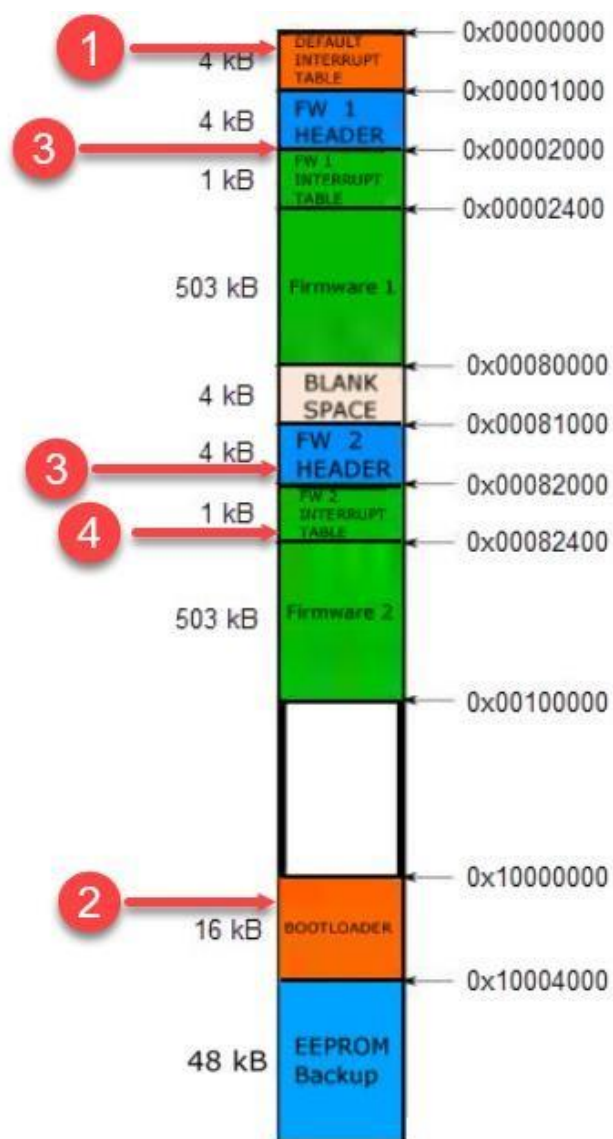
图14. S32K146引导过程
