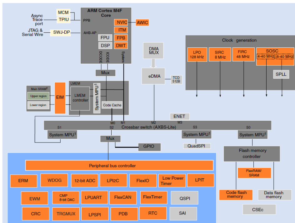
图7. S32K14x方框图
