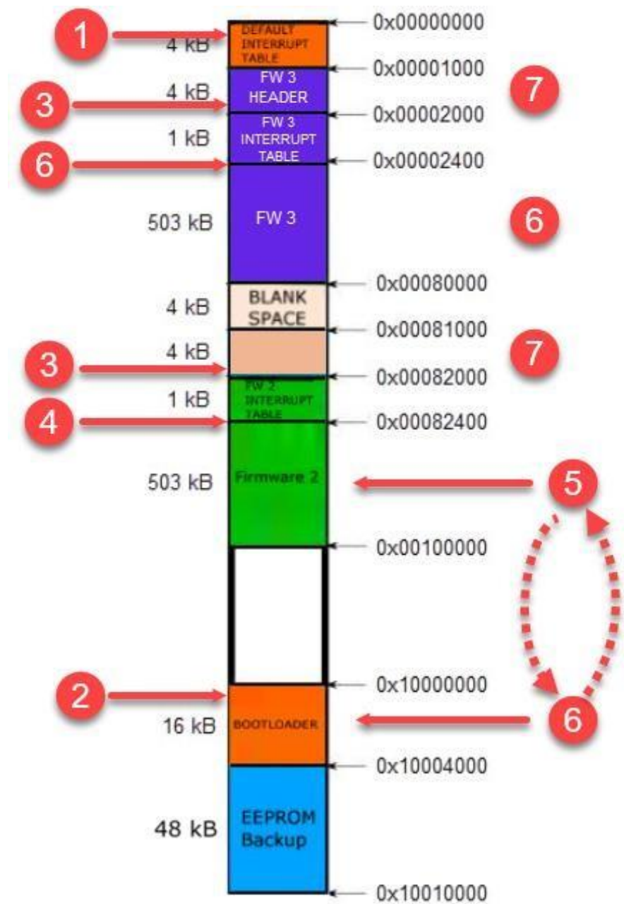
图16. S32K146更新过程 ( 场景2)
